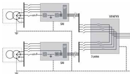
Figura 6: esquema de sistemas TNC
