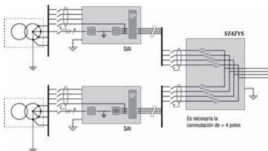
Figura 3: esquema de sistemas TT
