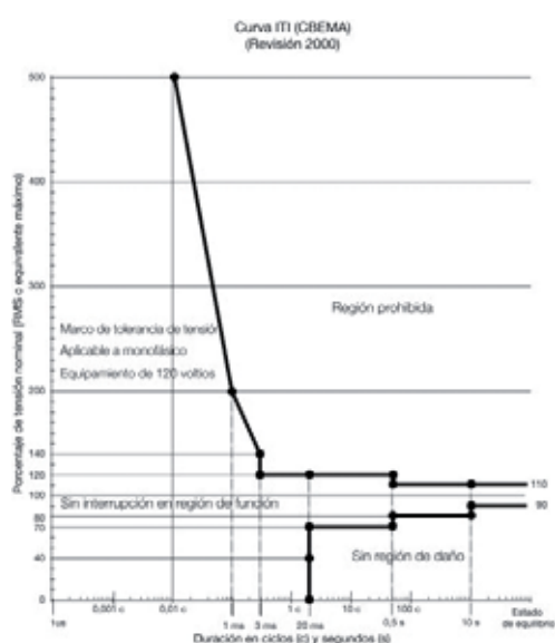
Figura 1: curva de ITIC
