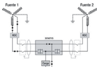
Figura 4: corrientes TT neutras sin conmutación de neutro
