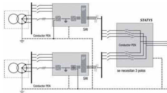
Figura 5: esquema de sistemas TNS
