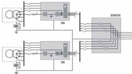
Figura 2: esquema de sistemas TI
